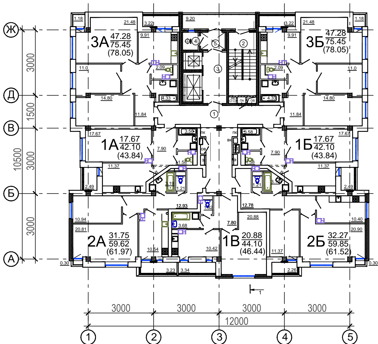
План типового этажа
