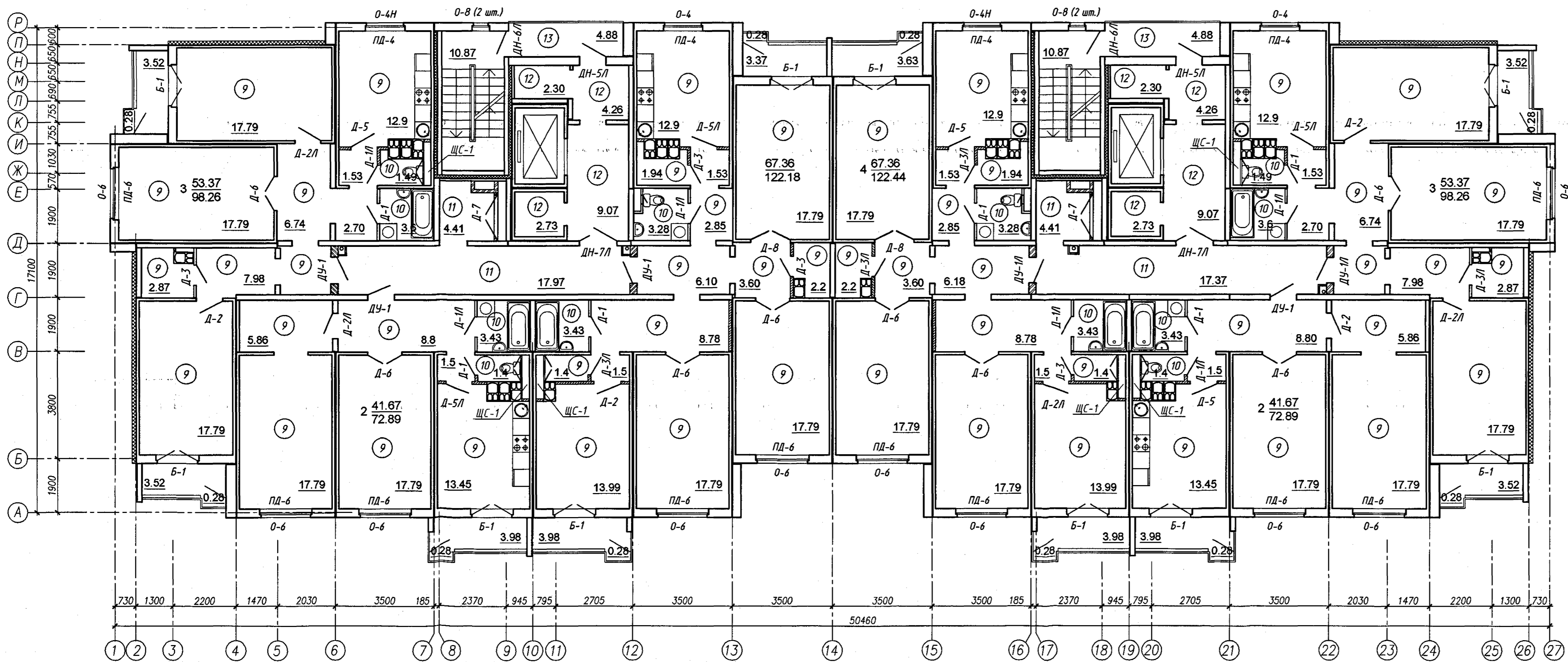
План 7-9 этажей
