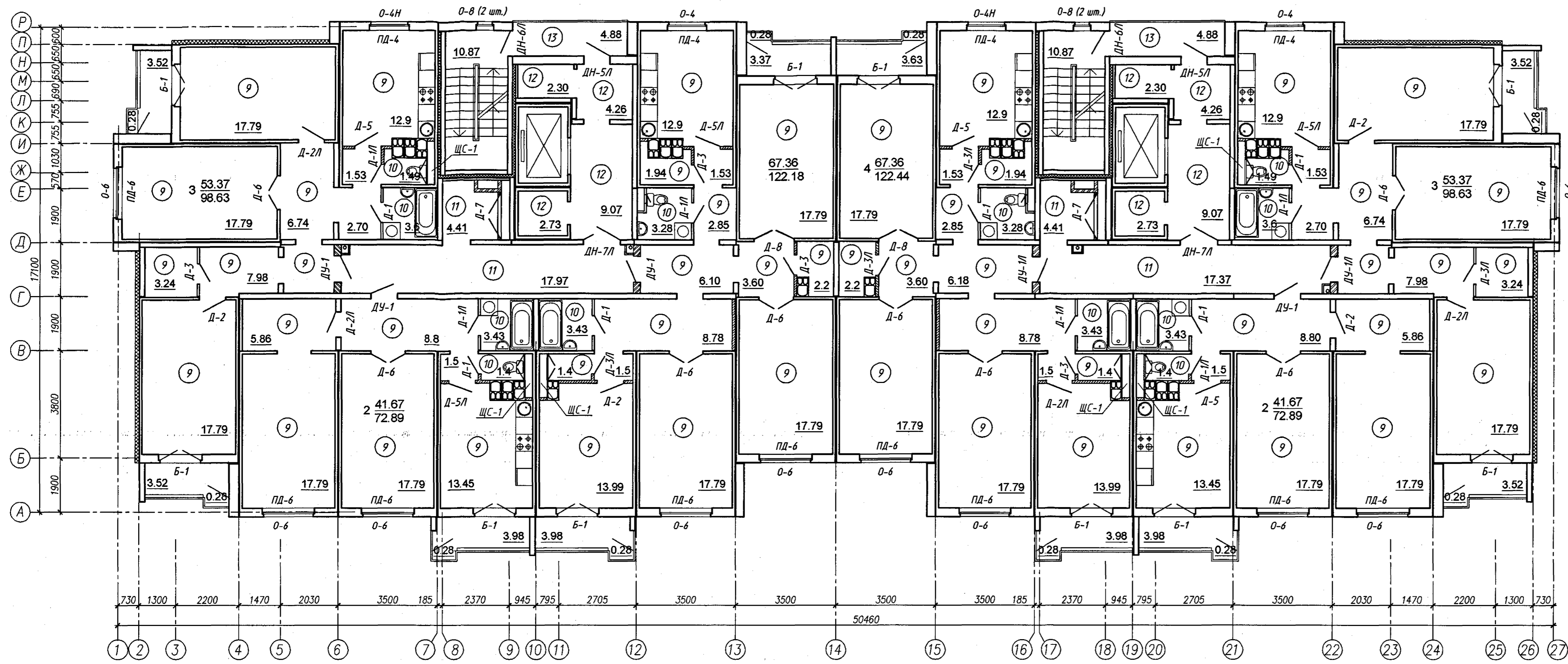
План 6-го этажа
